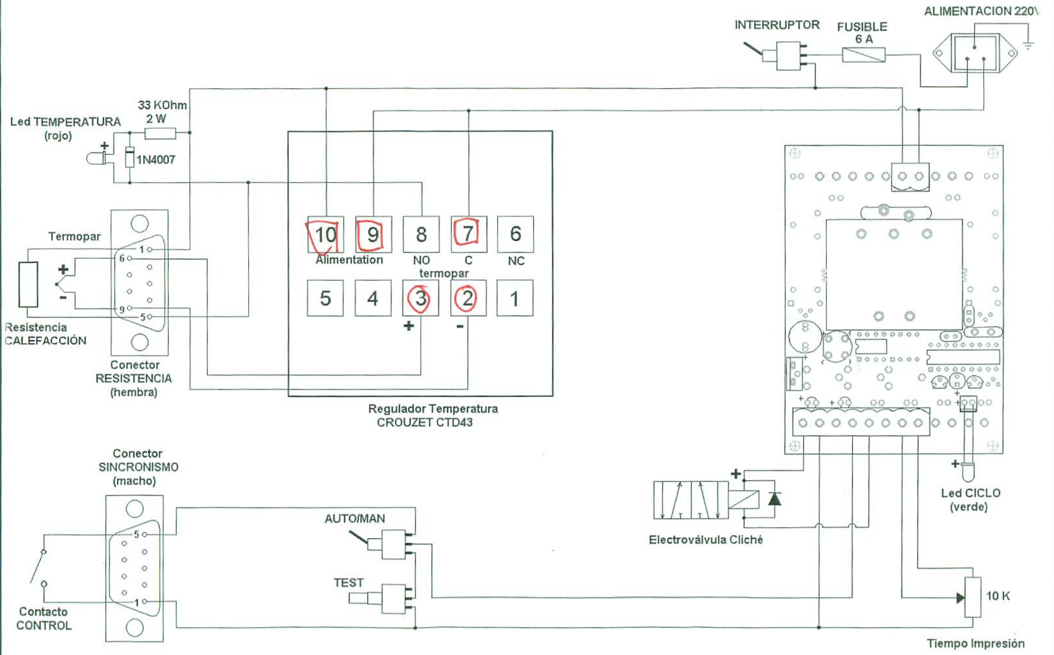
ESQUEMA CONEXIONADO EQUIPO TERMOIMPRESOR POR CLICHÉ
